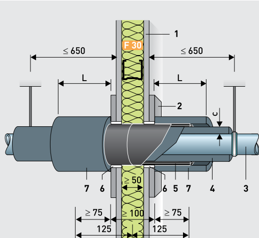
R 30-Abschottungen in einer leichte Trennwand F 30 nach DIN 4102-4 – Rohrinsolierung Synthetikgummi, Schaumglas
