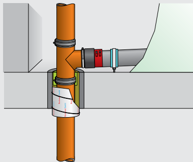
Rohr mit ROCKWOOL-Dämmstoffen = Körperschallentkopplung – Conlit Muffenrohrschale S – Steinwollestopfung – Conlit SML-Manschette
