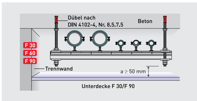
Rohrleitungsbefestigung oberhalb einer klassifizierten Unterdecke
