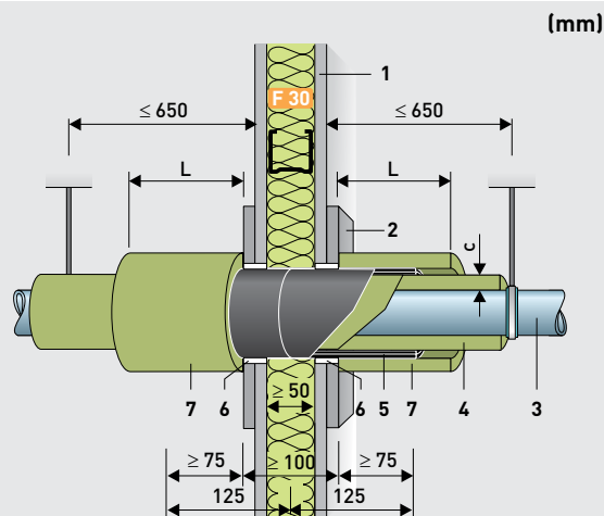
R 30-Abschottungen in einer leichte Trennwand F 30 nach DIN 4102-4 – Rohrinsolierung Mineralfaser A1/A2
