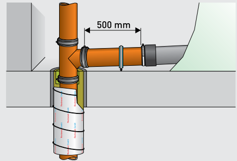
Rohr mit ROCKWOOL-Dämmstoffen = Körperschallentkopplung – Conlit Muffenrohrschale 500 mm – Steinwollestopfung
