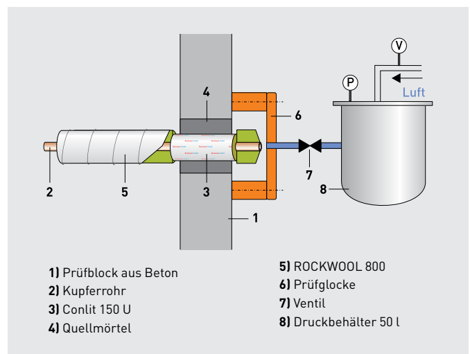
Prüfaufbau mit eingemörteltem isoliertem Kupferrohr
