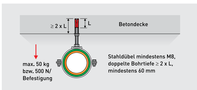
Nichtbrennbare Aufhängung nach DIN 4102-4, Nr. 8.5.7.5
