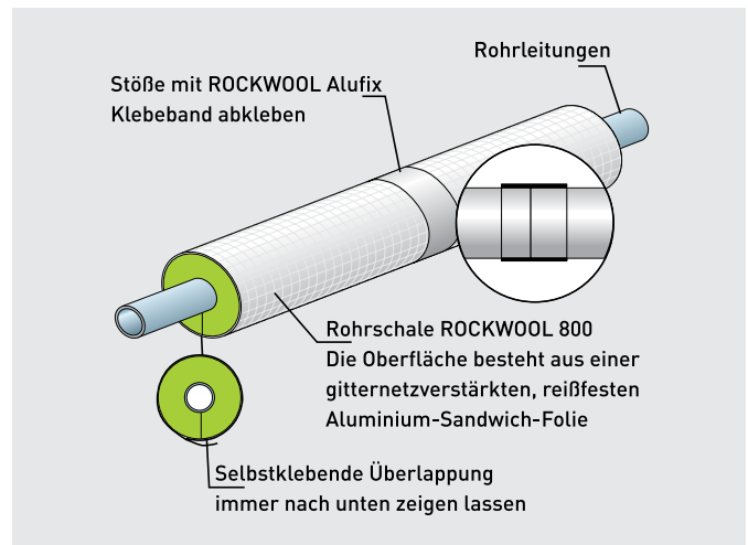
Abkleben der Rundstöße bei der ROCKWOOL 800
